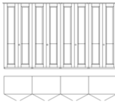
8-delna garderobna omara Šifra: 1280 ŠxVxG: 380 (390*) x 222 x 60
