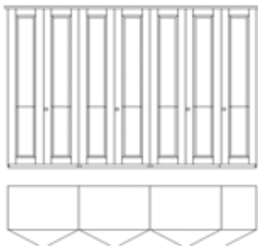
7-delna garderobna omara Šifra: 1270 ŠxVxG: 319 (329*) x 222 x 60
