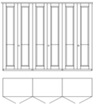
6-delna garderobna omara Šifra: 1260 ŠxVxG: 275 (285*) x 222 x 60
