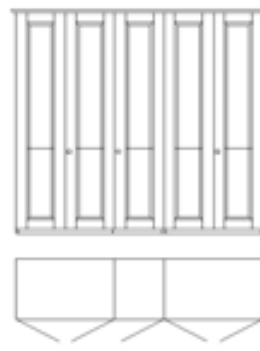
5-delna garderobna omara Šifra: 1250 ŠxVxG: 229 (239*) x 222 x 60
